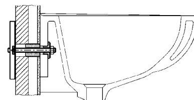
Mosdó rögzítés billenő dübellel M10
